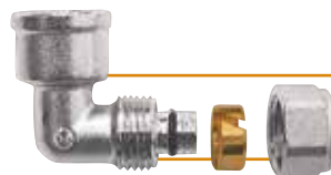
COUDE FEMELLE
