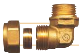
COUDE MÂLE
