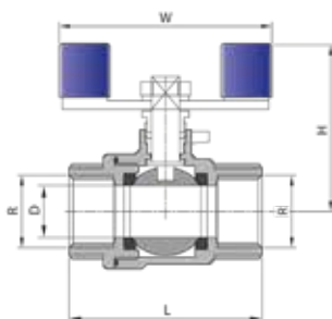
VANNE À SPHÈRE 2 PIÈCES
